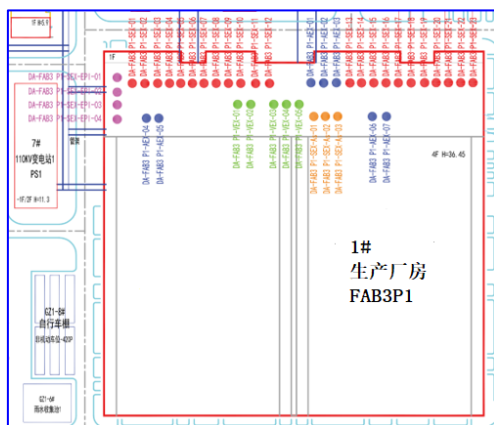
图 1 酸、碱、有机、酸性含砷、酸性外延废气监测点位图
